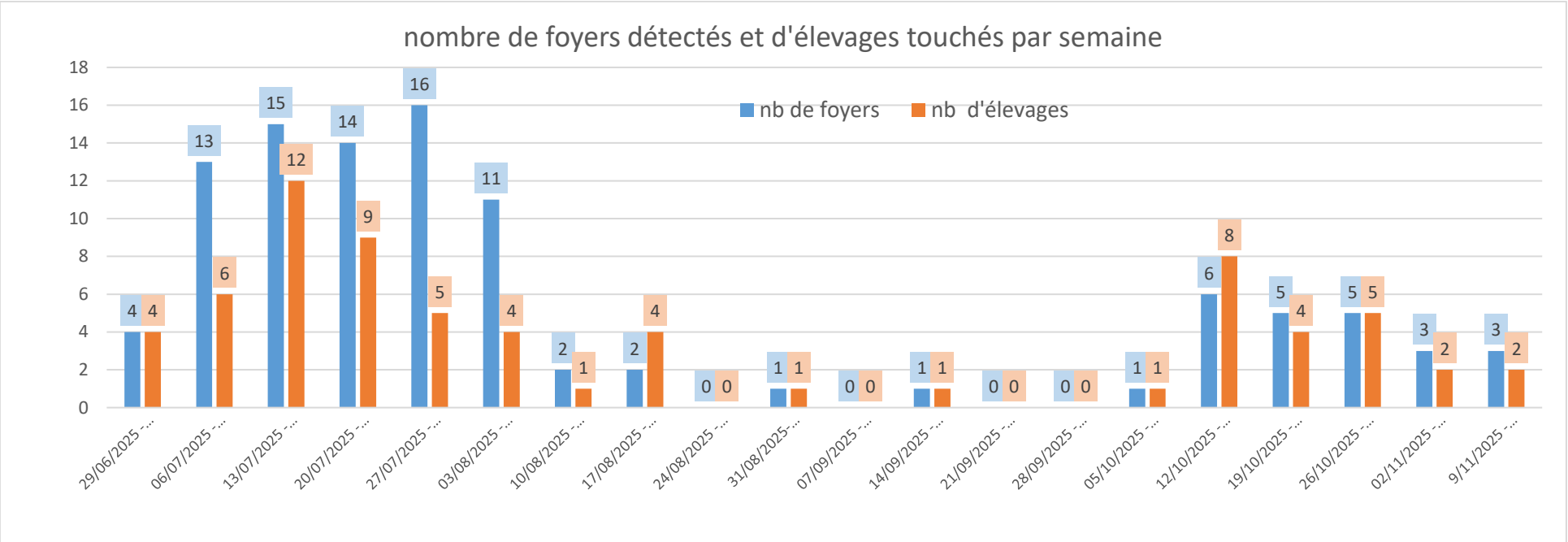
Figure 1 : Évolution hebdomadaire du nombre de foyers de DNC et d'élevages 1 touchés depuis le 29/06/2025 (selon date de confirmation)
